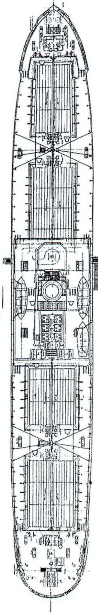
— Vue en Plan —
